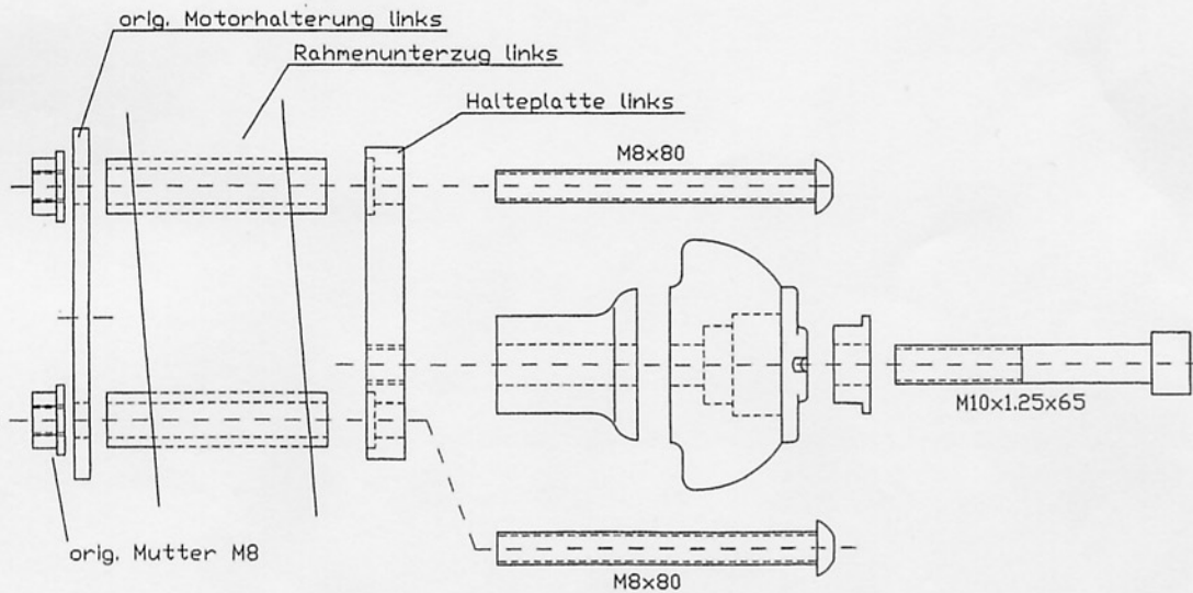
Montagetelle links, Ansicht von vornel
