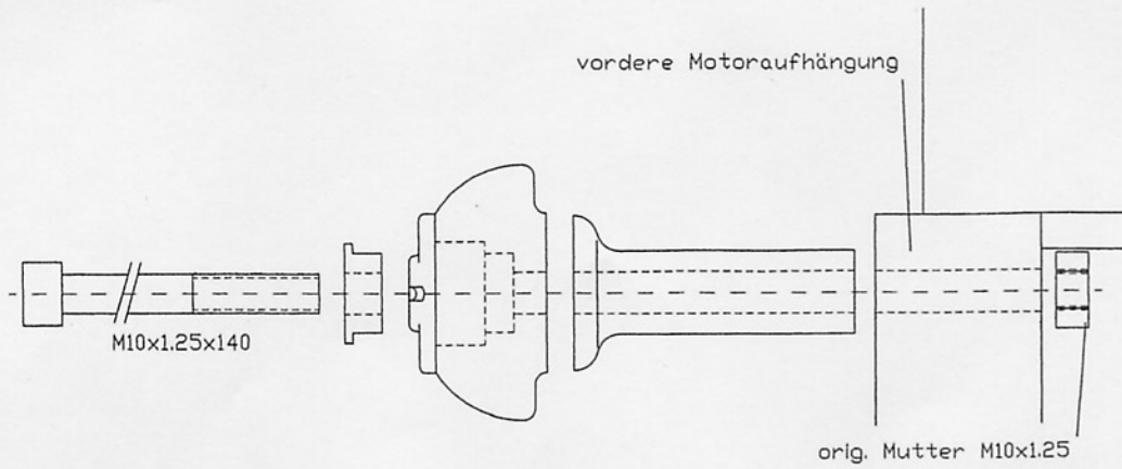
Montagetelle rechts, Ansicht von vornel
