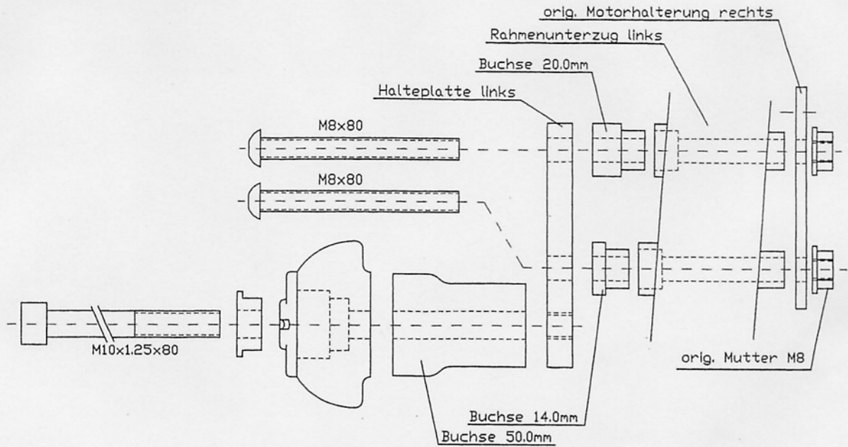
Montageteile rechts, Ansicht von vorne!
