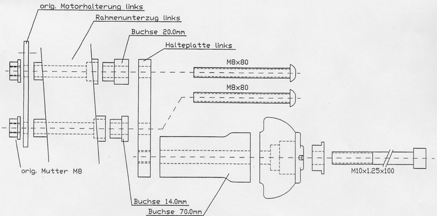
Montageteile links, Ansicht von vorne!
