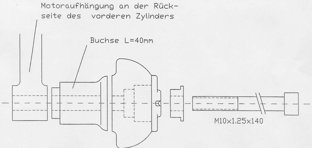
Montageteile links, Ansicht von vorne!
