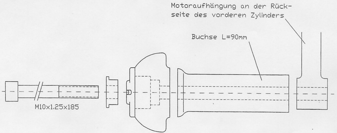
Montageteile rechts, Ansicht von vorne!
