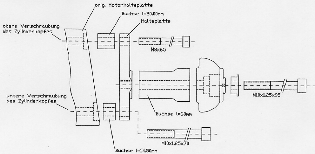
Montagetelle rechts, Ansicht in Fahrtrichtung
